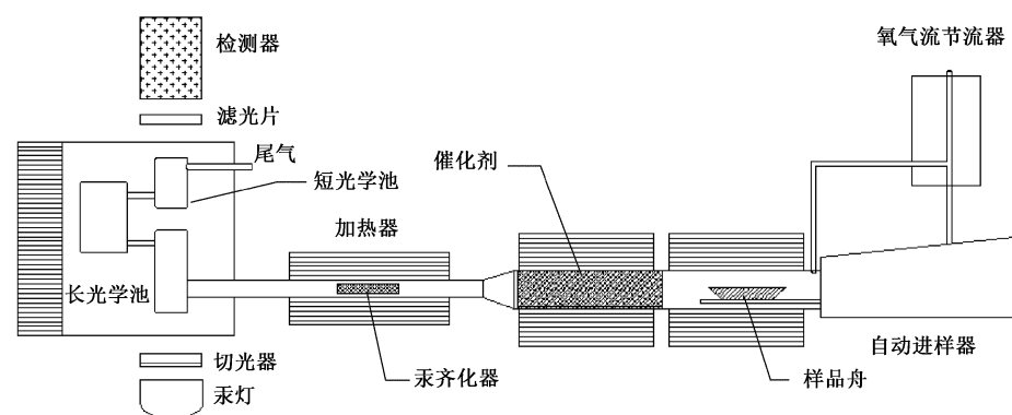
图 A.1 直接测汞仪原理图
